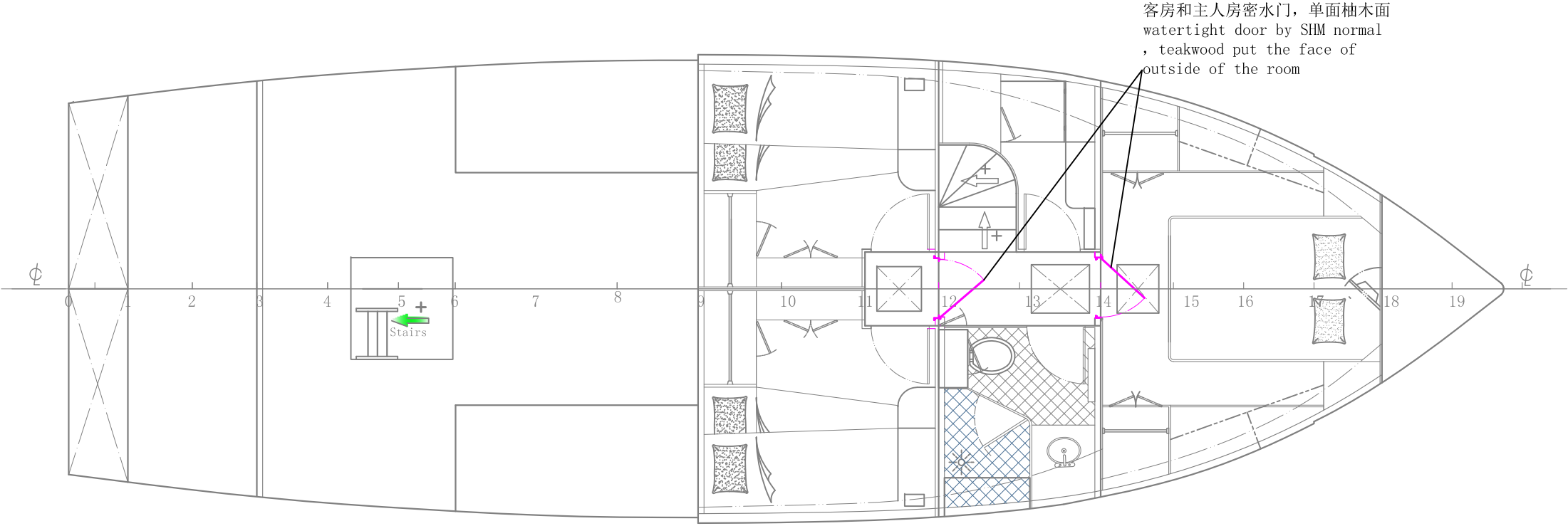
46207船 门窗标示图 SD46207 Door and Windows
