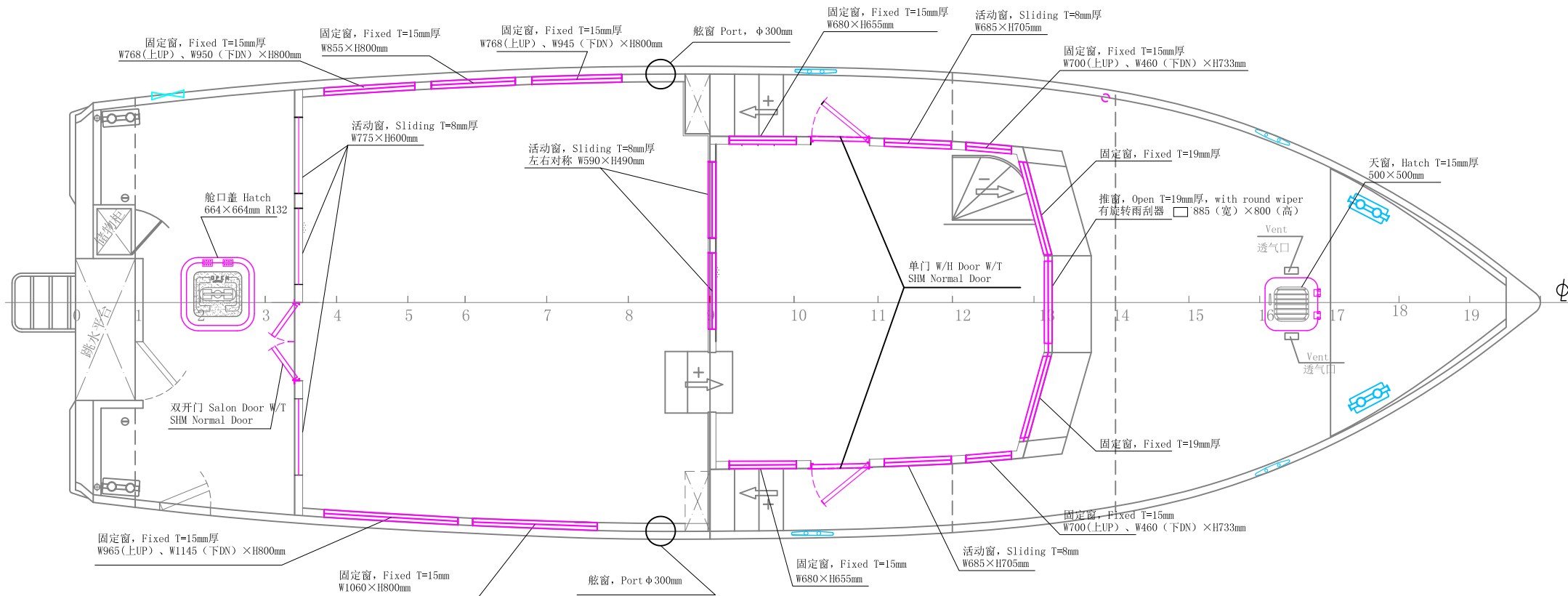
46207船 门窗标示图 SD46207 Door and Windows
