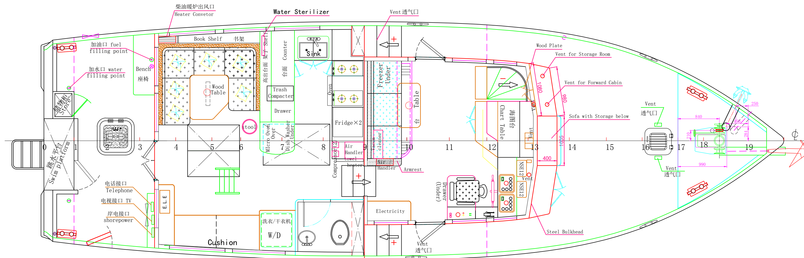
甲板平面图 Main Deck Plan
